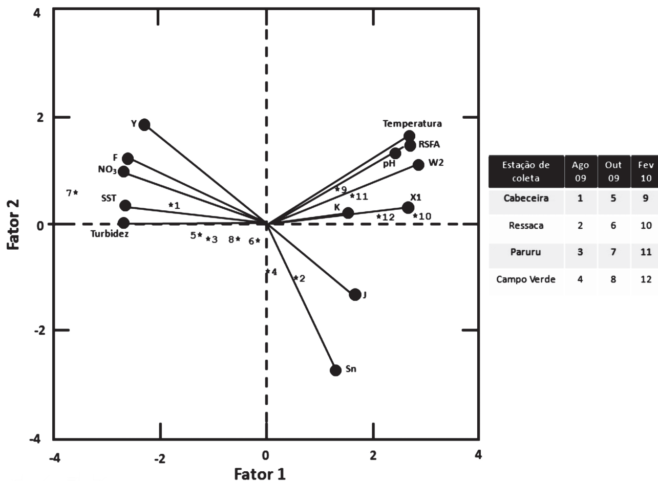
Figura 5. Biplot dos componentes principais (Fatores 1 e 2). Os vetores plotados indicam os scores de correlação obtidos entre as variáveis da água (características físicas e químicas e grupos funcionais fitoplanctônicos) e os dois fatores. Os números no interior dos quadrantes se referem às estações amostrais no inverno (1 a 4), primavera (5 a 8) e verão (9 a 12).
