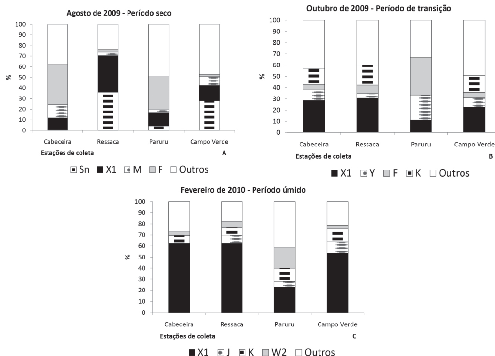
Figura 4. Principais grupos fitoplantônicos e sua abundância relativa no reservatório de Ituparanga em agosto (A) e outubro (B) de 2009 e fevereiro (C) de 2010, de acordo com a classificação fitossociológica de Reynolds.
