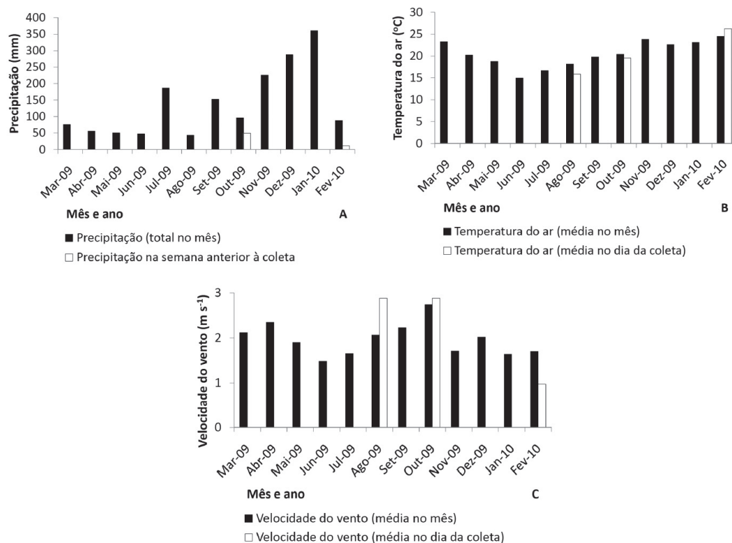
Figura 2. Dados climatológicos da área de estudo nos anos de 2009 e 2010: precipitação pluviométrica (A), temperatura do ar (B) e velocidade do vento (C). Para cada variável, são apresentados os totais ou as médias referentes ao mês e aos dias de coleta ou à semana antecedente.
