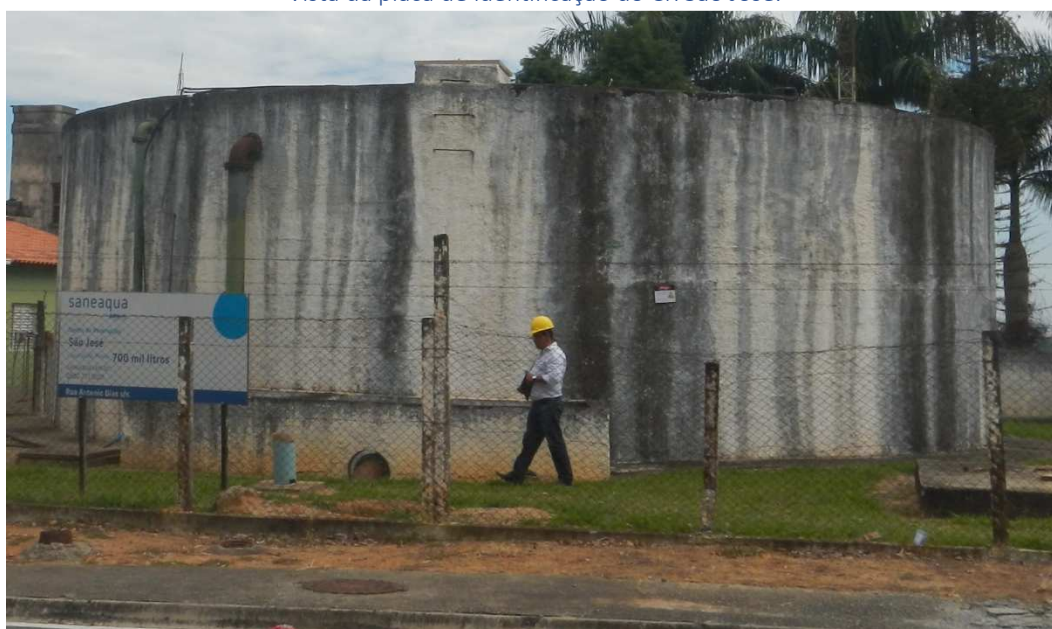
Vista do Reservatório pertinente ao CR São José com capacidade de 700 m 3 .
